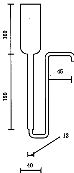
图2 离子交换柱
