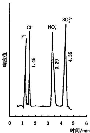
图 1 离子色谱图
